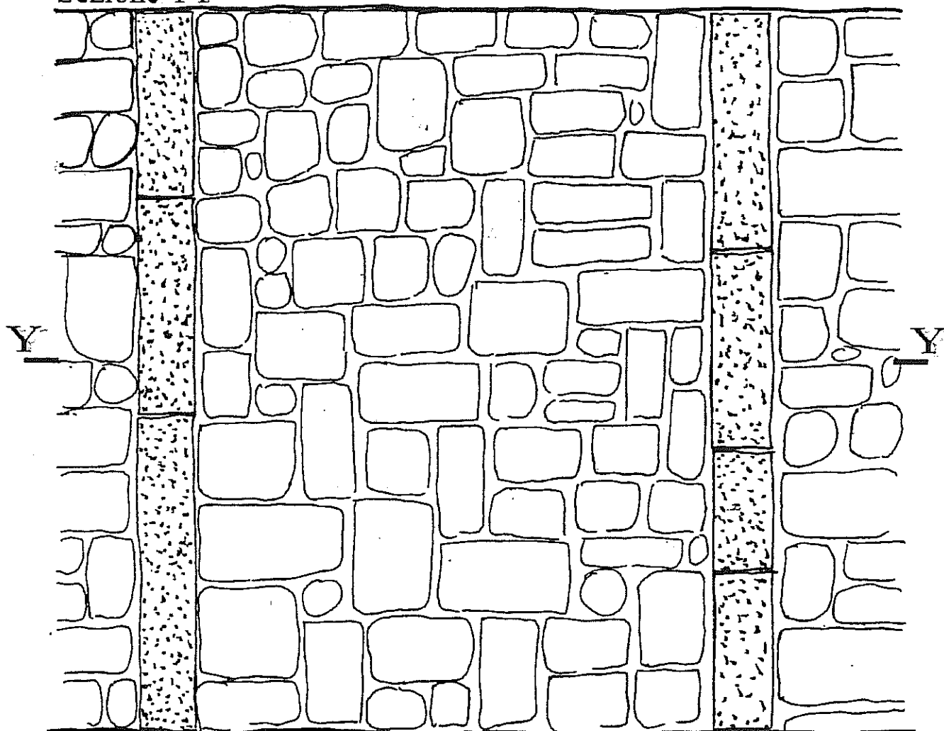
Pianta
