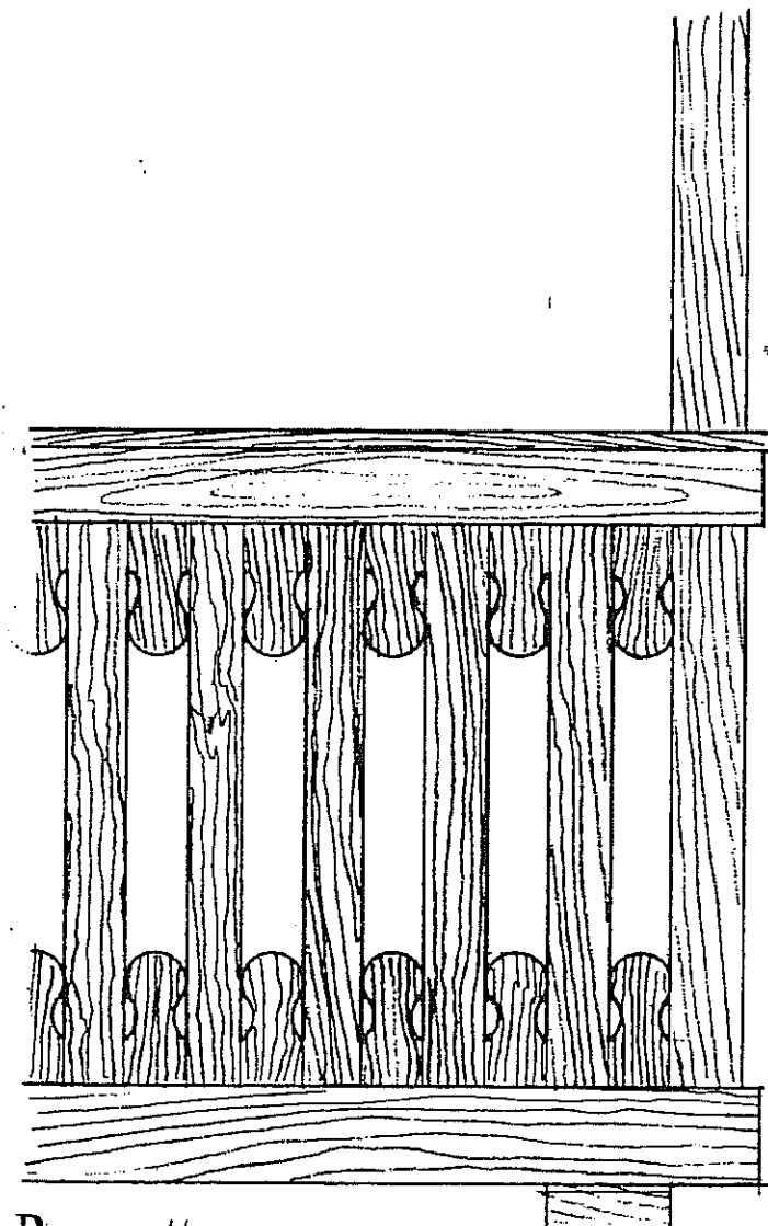
Prospetto
